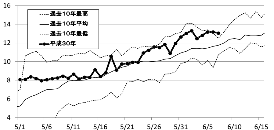
平成30年サロマ湖水温(中央部)
